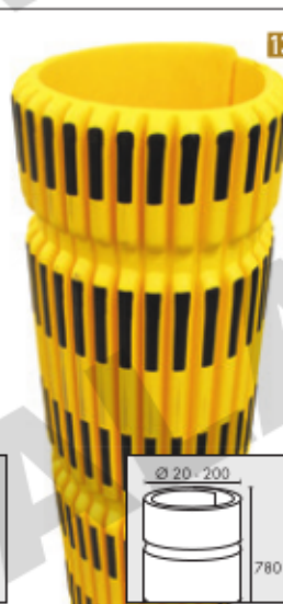
8 PGE230S - paracolpi lunghezza 780 mm x larghezza 28 mm, peso 135 gr senza biadesivo
