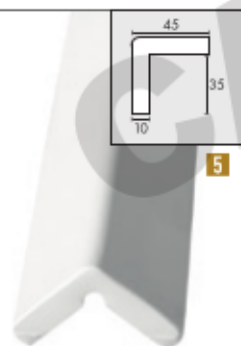
5 PGE320SW - paracolpi lunghezza 780 mm x 45 mm, peso 135 gr con biadesivo, colore bianco PGE320SWM - come sopra ma magnetico
