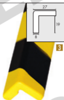
3 PGE320S - paracolpi lunghezza 780 mm x larghezza 27 mm, peso 135 gr con biadesivo PGE320SM - come sopra ma magnetico
